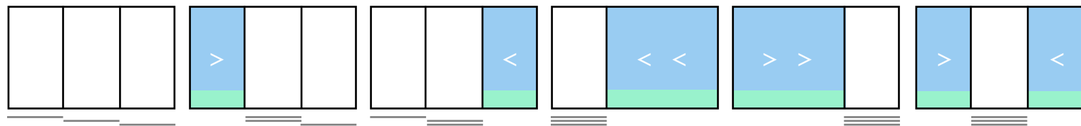
Le possibilità di apertura di Tecnocor>2 nella sua versione a tre ante.
